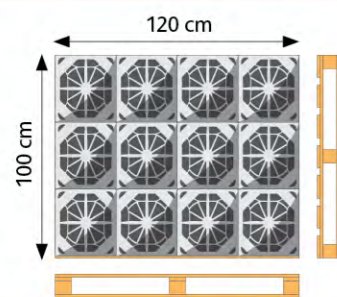
Blokpallet - 12 containers per laag
