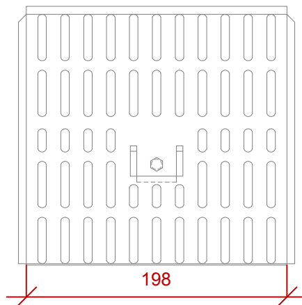
Opstalt C-C 1:4
