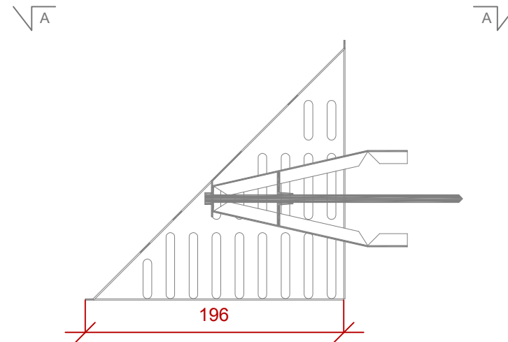
Snit B-B 1:4
