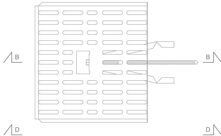
Plan A-A 1:4
