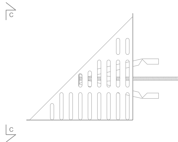
Opstalt D-D 1:4
