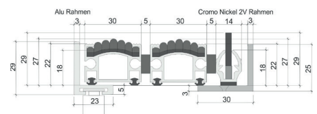
Alumatte Classic - Rips und Bürste 2:1 Höhe 27 mm
