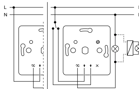
Девиатор – ERH66001xx
