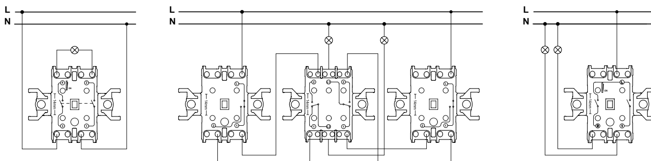
Двуполюсен ключ
