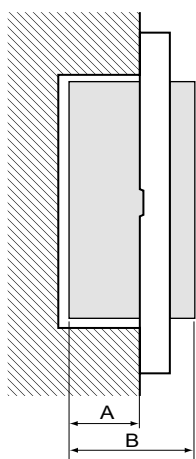
A: Дълбочина на вграждане B: Дълбочина на механизма
