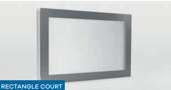
RECTANGLE COURT Entourage : 534 x 344 mm Clair de vitrage : 452 x 262 mm
