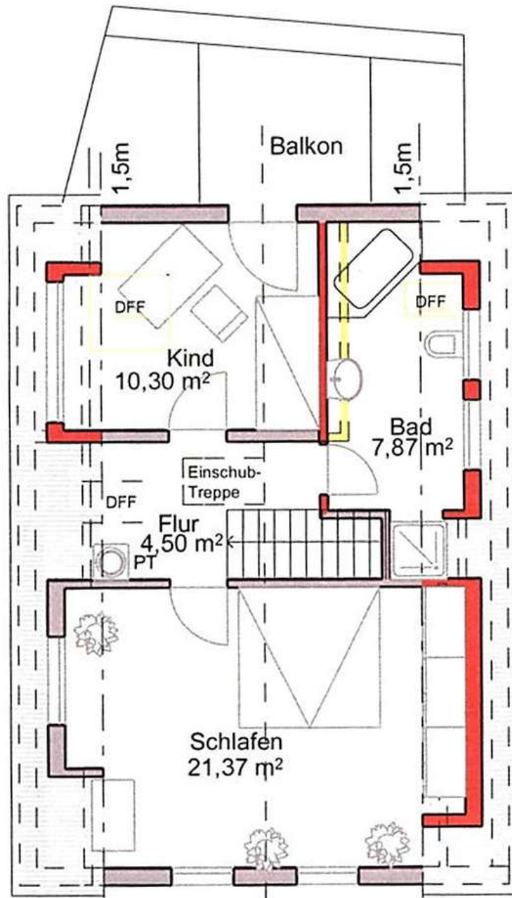
Dachgeschoss
