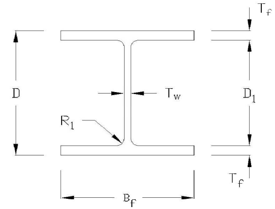
UNIVERSAL COLUMNS
