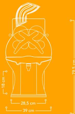
Vorderansicht
